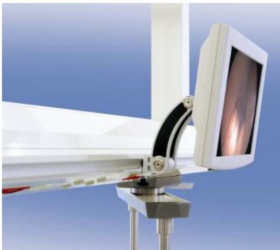
Soporte monitor TFT sobre raíl
